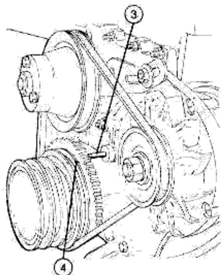
3. Indice fisso 4. Tacca puleggia
