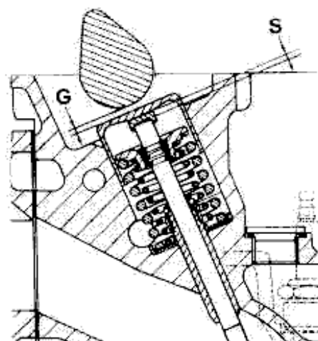
G. Gioco valvola S. Spessore cappellotto di regolazione
