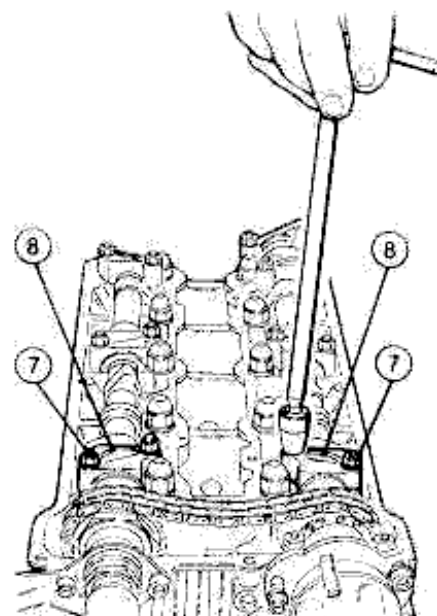
7. Dadi fissaggio cappelli 8. Cappelli alberi distribuzione
