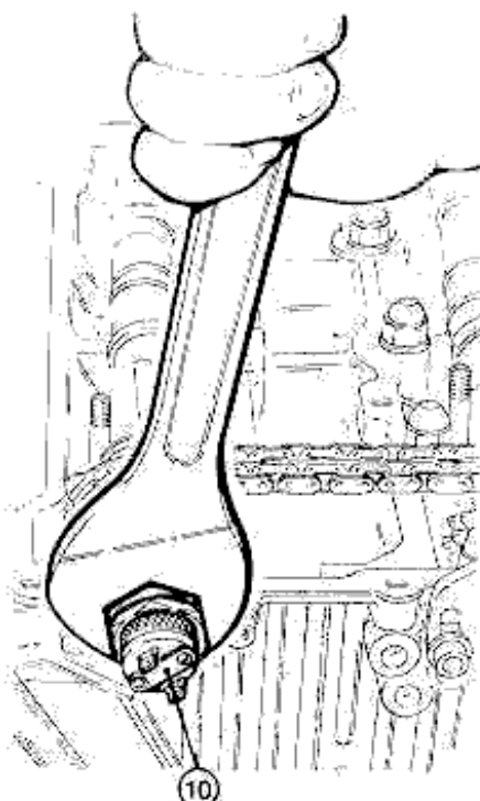
10. Elettromagnete variatore di fase
