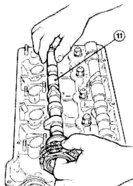
11. Albero distribuzione lato aspirazione
