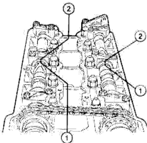
1. Tacche alberi distribuzione 2. Tacche cappelli
