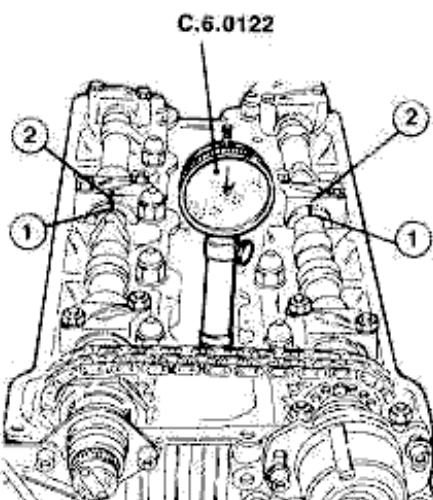
1. Tacche alberi distribuzione 2. Tacche cappelli
