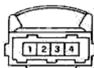
CONNETTORE MODULO BOBINA B - VISTA FRONTALE
