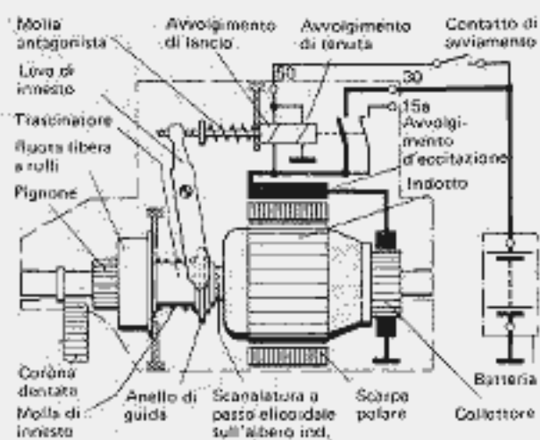
Rappresentazione schematica del motorino a traslazione ed avvistamento del pignone.
