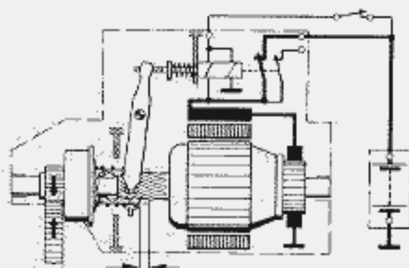
Trascinatore mosso dalla rotazione dell'indotto (avvita-mento) / Il motore viene posto in rotazione.
