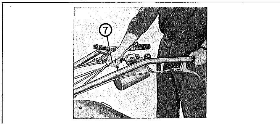
Fig. 5 - Bloccaggio differenziale
