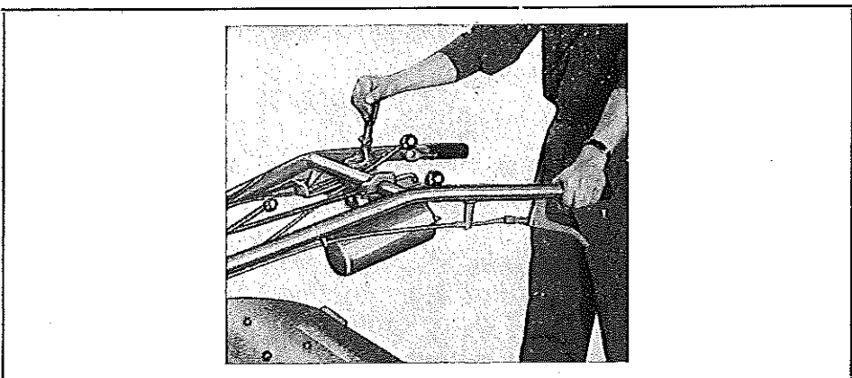
Fig. 8 - Frenata simultanea
