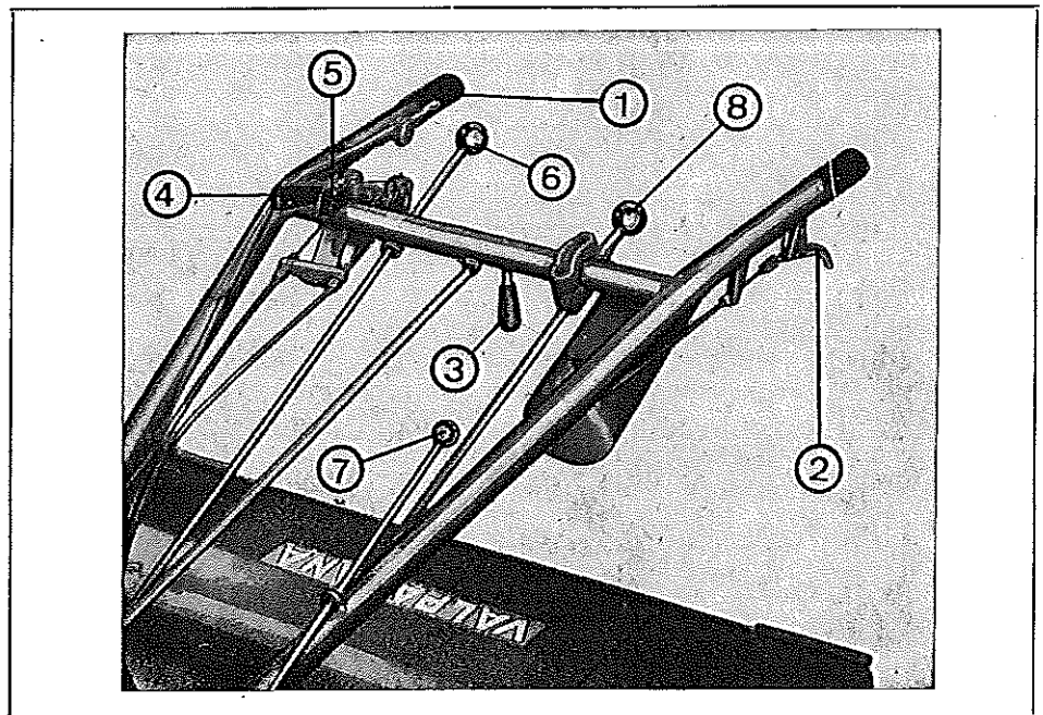
Fig. 1 - Disposizione comandi
