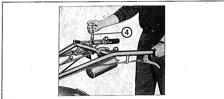
Fig. 6 - Frenata ruota destra
