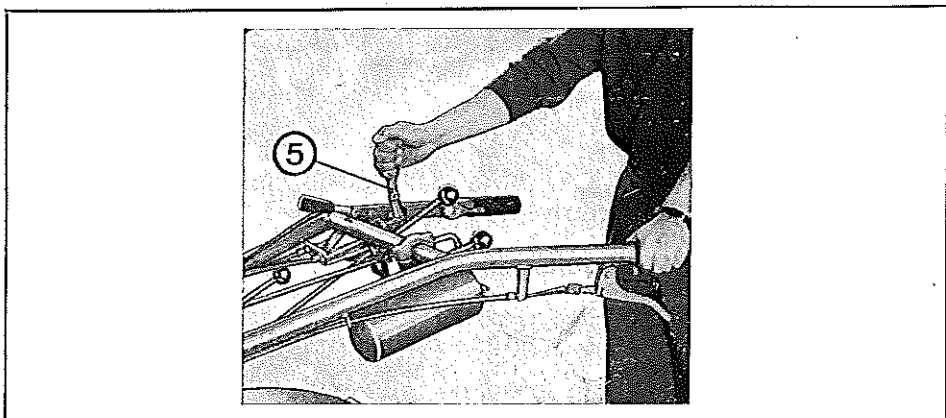
Fig. 7 - Frenata ruota sinistra
