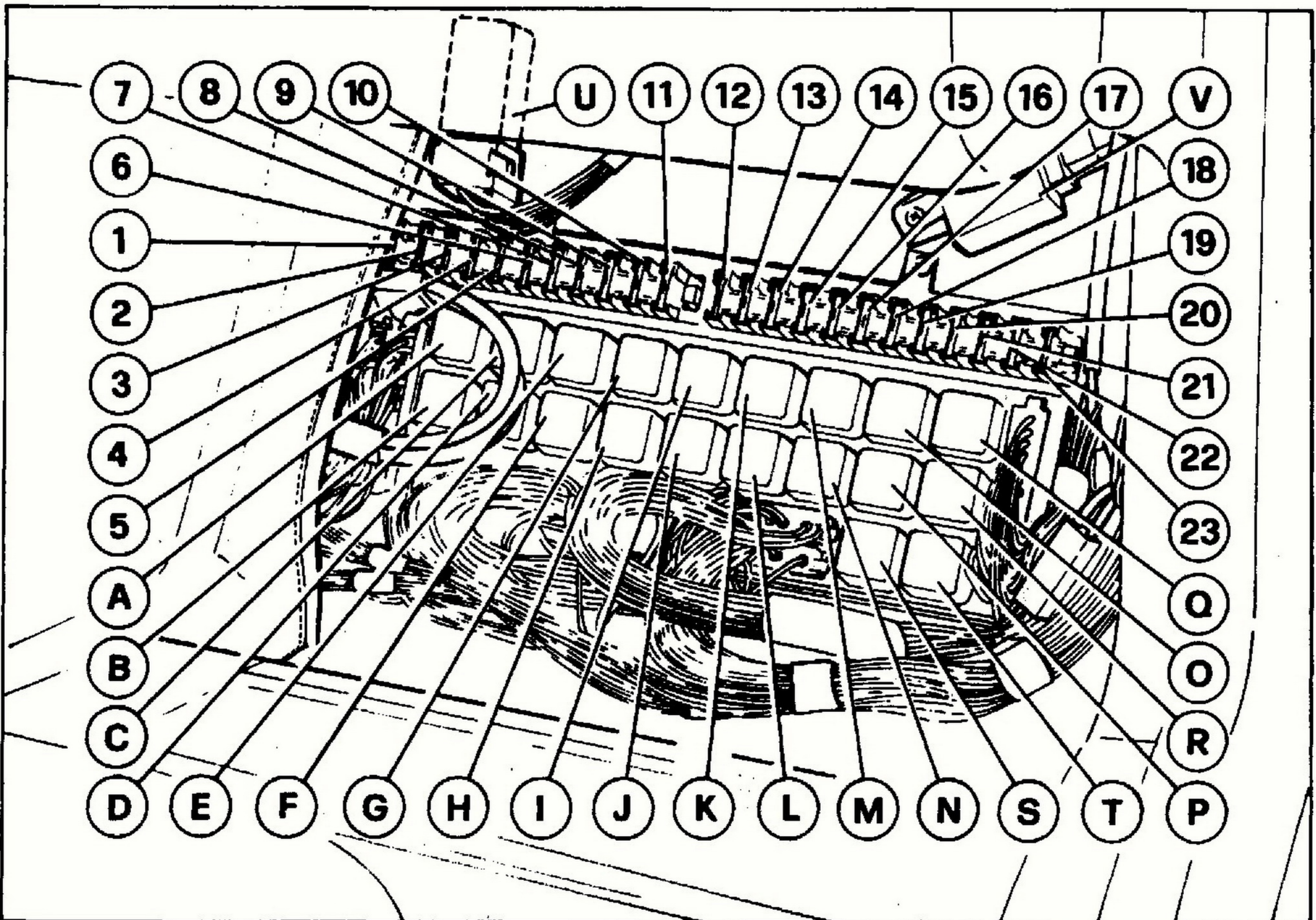
77) Valvole fusibili e teleruttori
