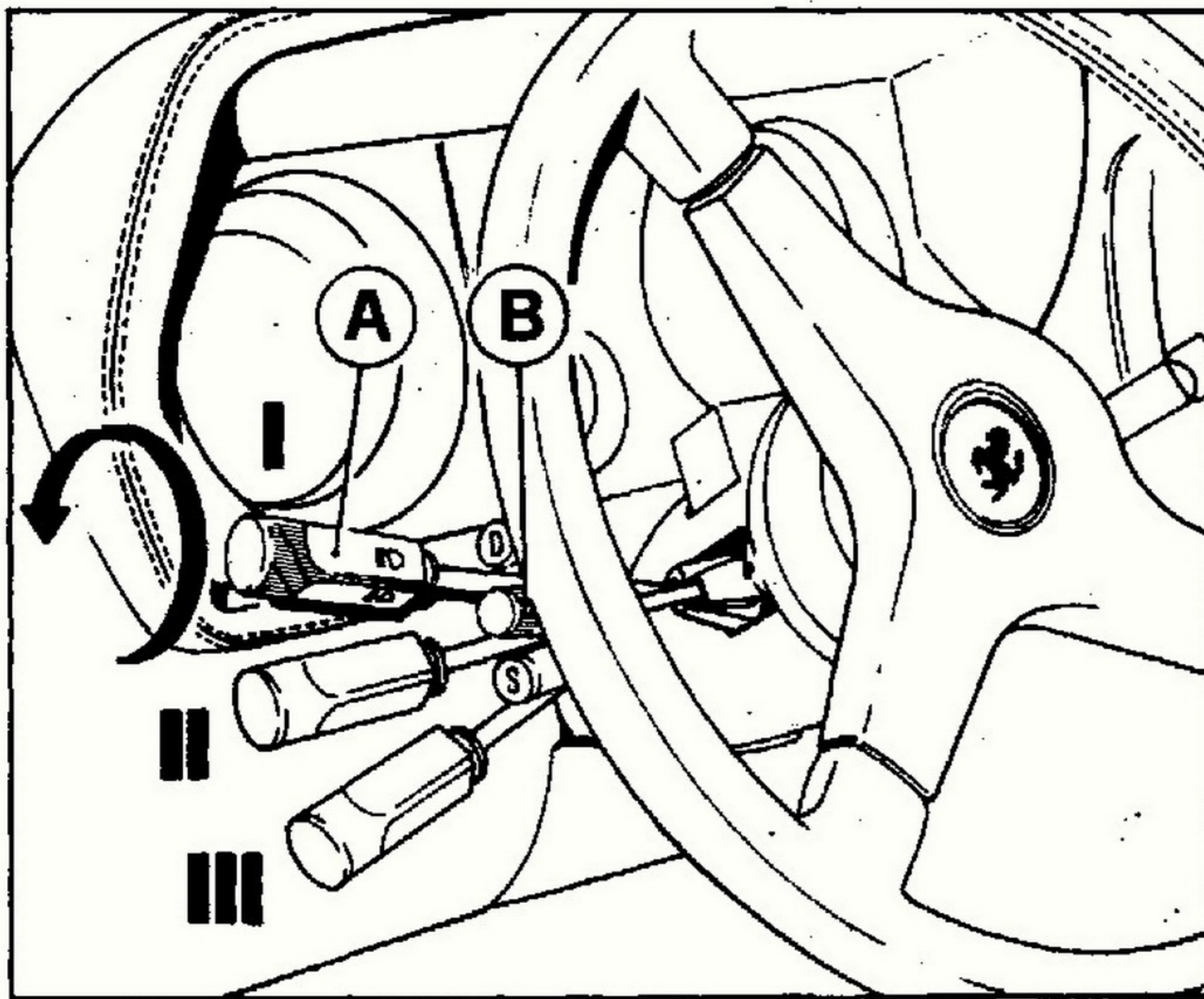
10) Leve di commutazione. 10) Combinateur d'éclairage phares et clignoteurs de direction. 10) High/low beam and direction indicator control levers.
