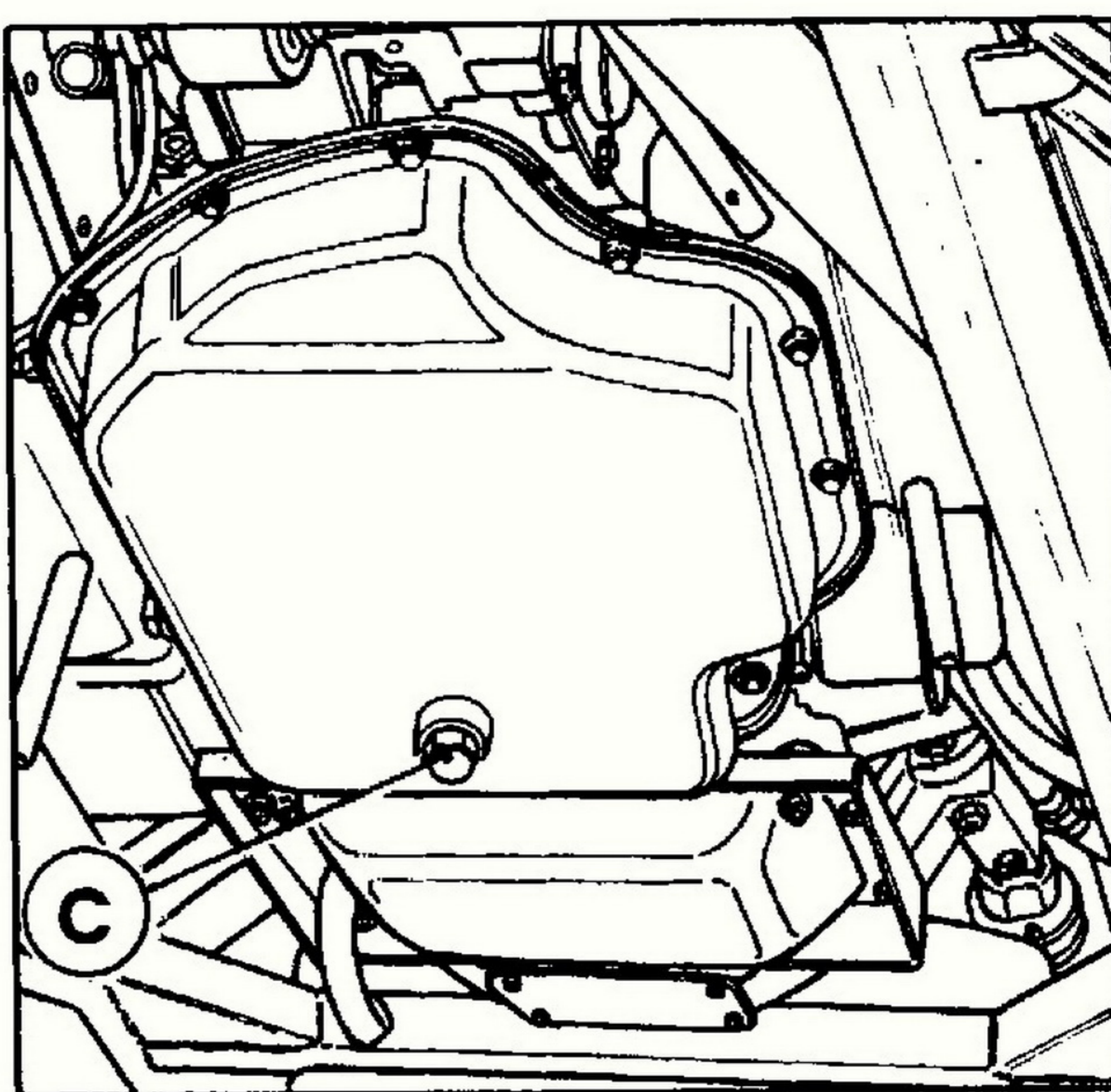
56) Sostituzione olio cambio automatico C - Coperchio inferiore cambio.
