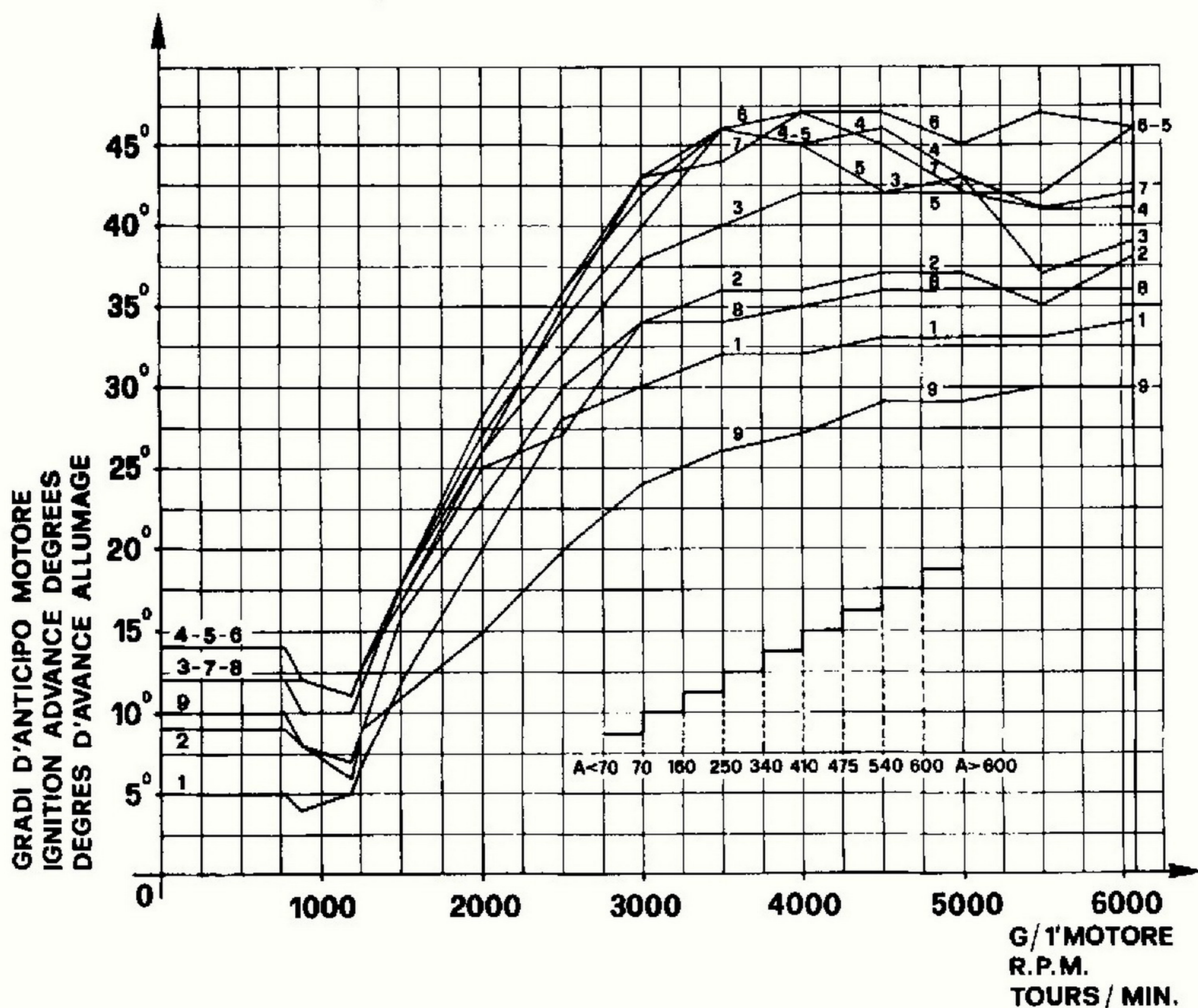
53) Courbe de l'avance
