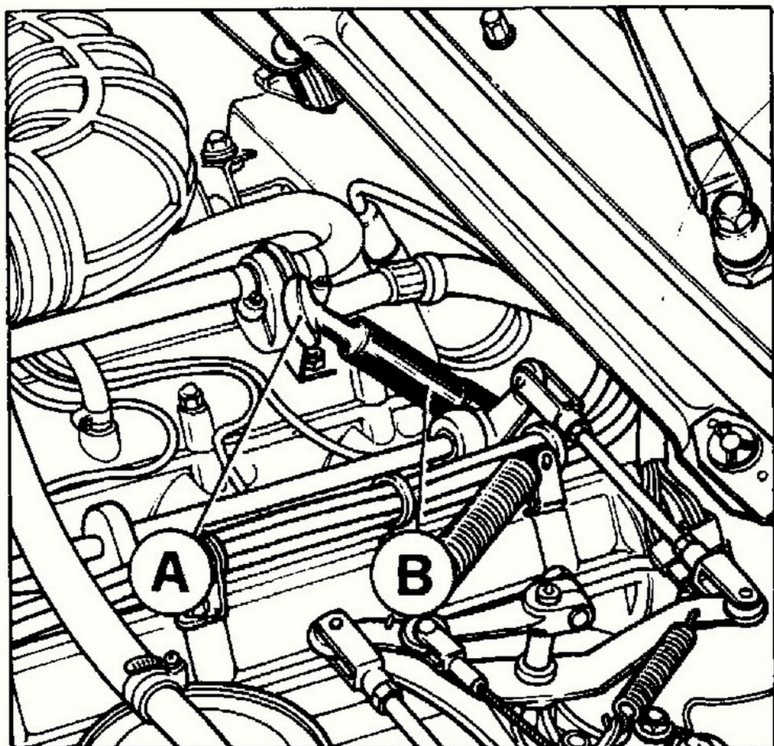
55) Asta livello olio cambio automatico A - Asta livello; B - Tubo asta livello e carico olio.
