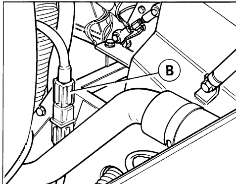
72) Posizione staccabatteria
