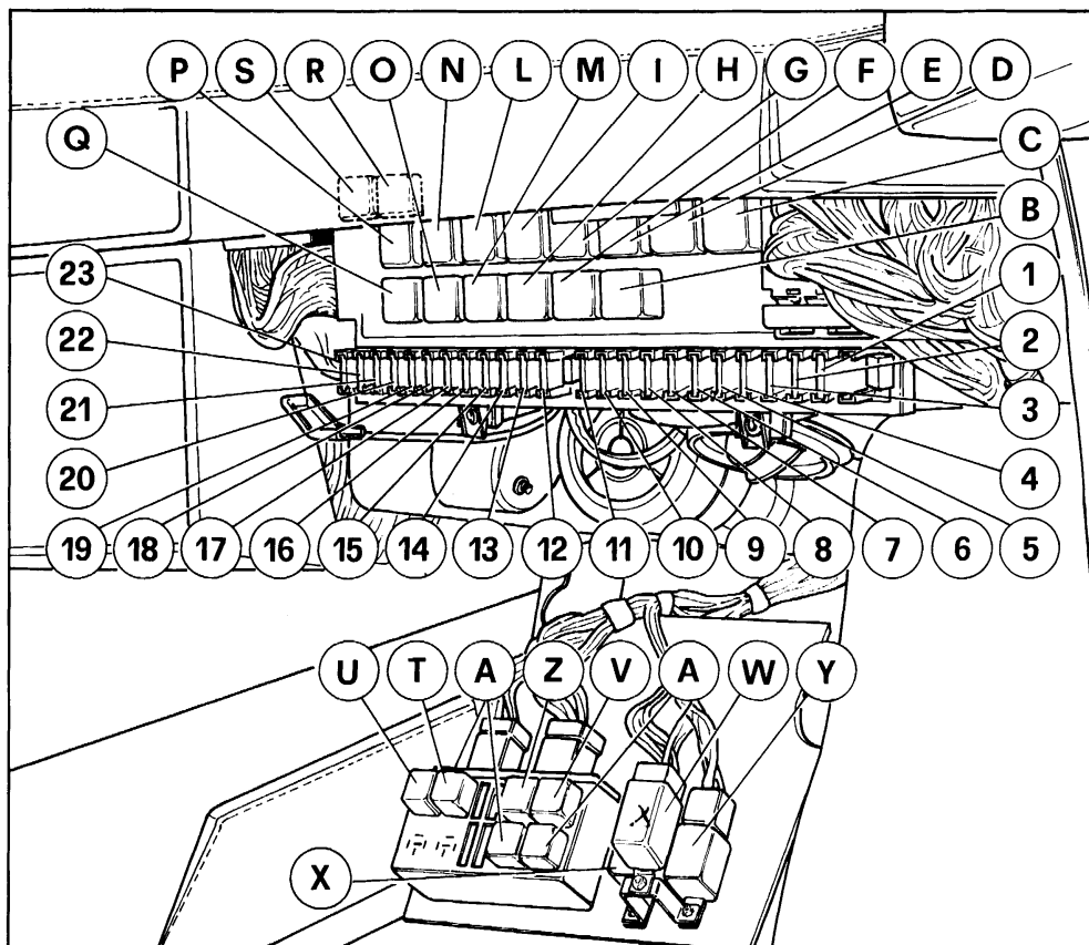
79) Valvole fusibili e teleruttori
