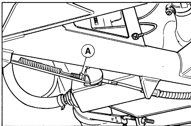
70) Regolazione freno a mano A - Dado di registro
