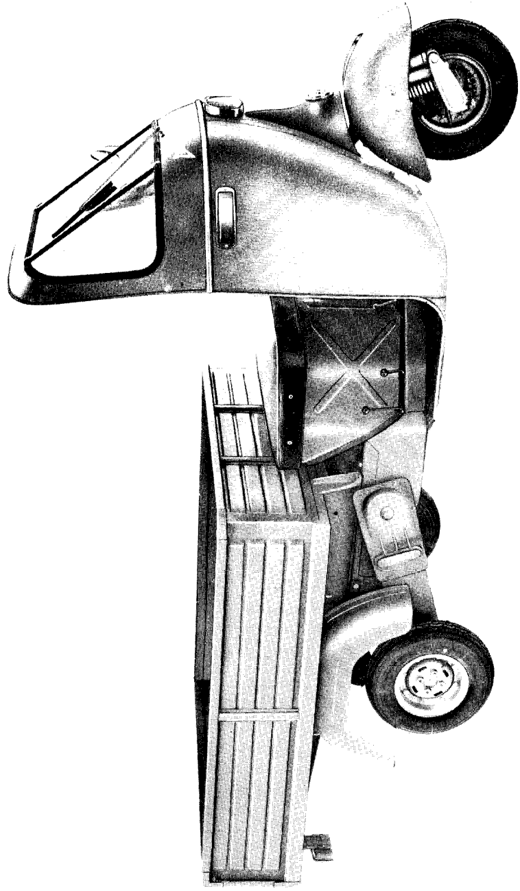
Fig. 4 - Motocarro con pianale e parasole
