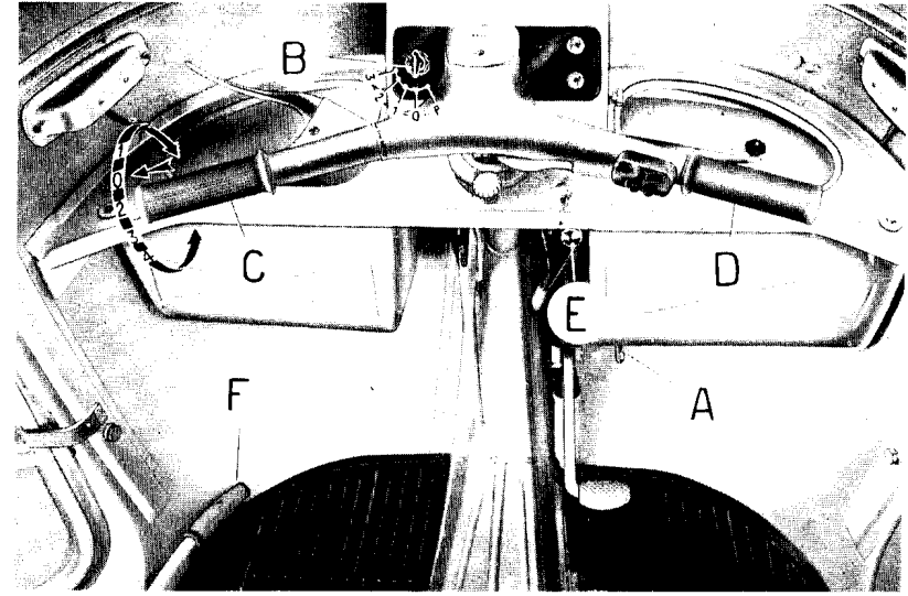
Fig. 10 - Coperazioni per avviare il motore
