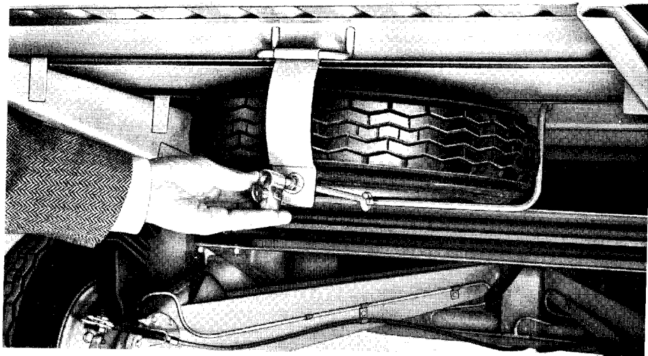
Fig. 16 - Fissaggio ruota scorta nel cestello
