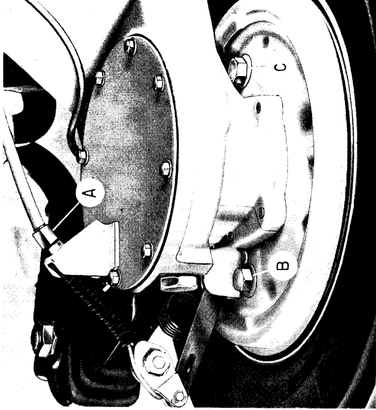
Fig. 20 - Registrazione freni posteriori, meccanici (registro a vite « A ») e idraulici (dadi « B » e « C »).
