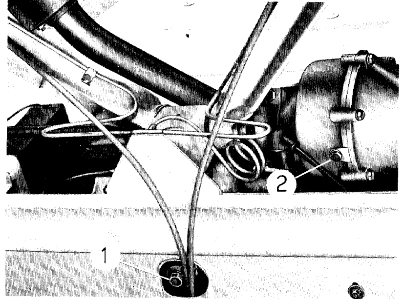
Fig. 22 - Fori di scarico olio dal motore, sotto il telaio, (1) e dal differenziale (2)
