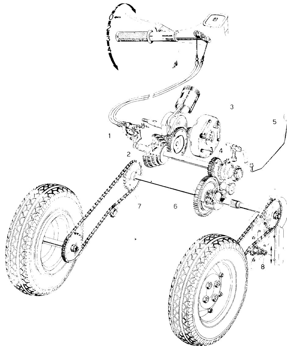
Fig. 12 - Schema del cambio e trasmissione alle ruote posteriori
