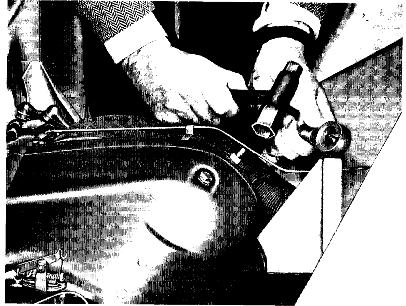
Fig. 21 - Smontaggio candela
