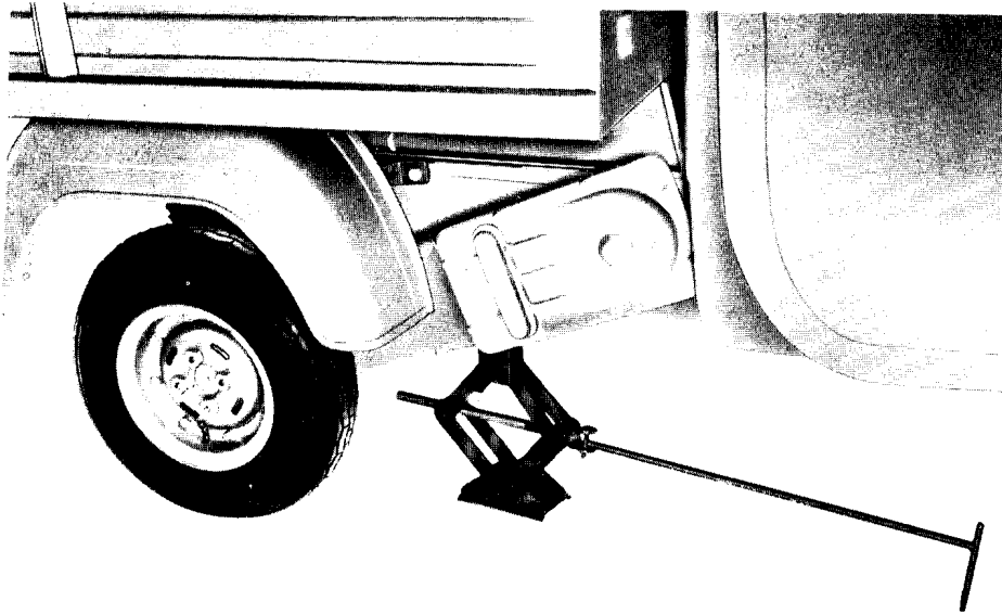
Fig. 15 - Applicazione martinetto di sollevamento - Smontaggio ruota.
