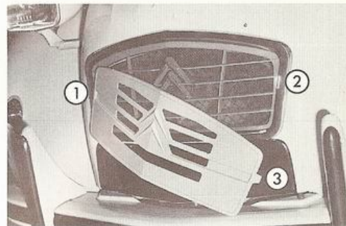
Fig. 23 - Applicazione della mascherina 1 - 3 - Linguette di fissaggio 2 - Alloggiamenti di fissaggio
