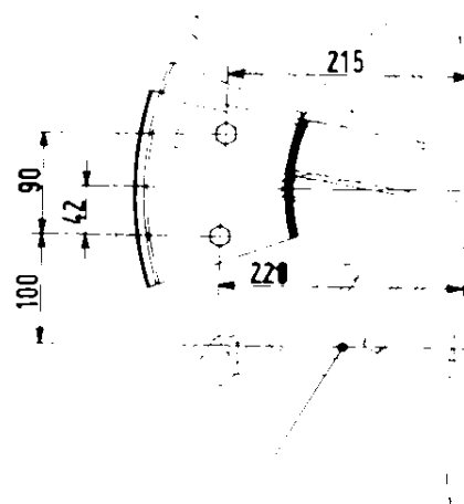
Mezzeria vettura
