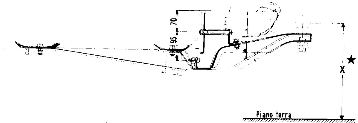
Sezione A-A
