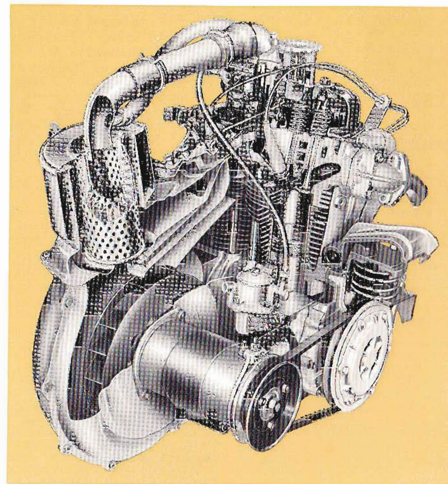
Motore con ventilatore, sezionati parzialmente
