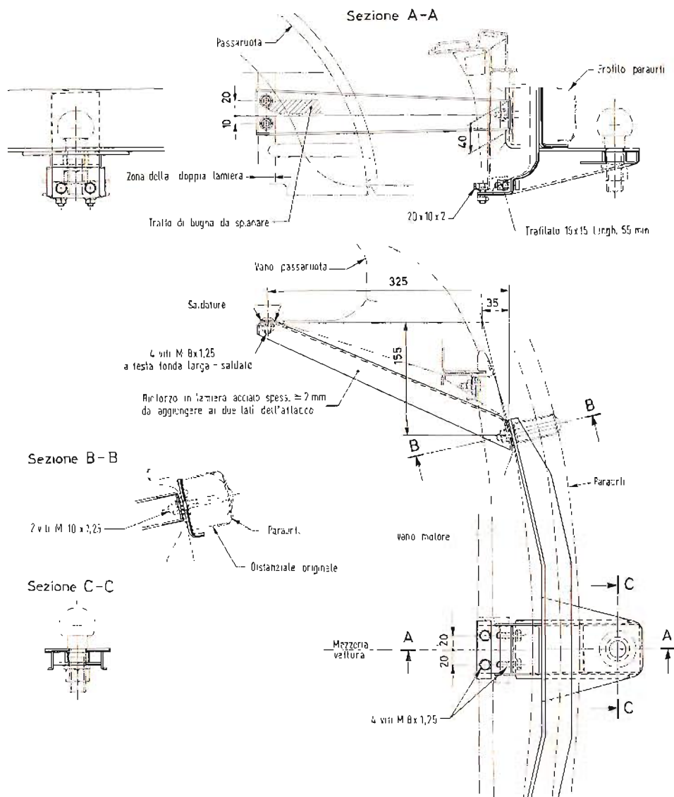
Installazione attacco traino rimorchio
